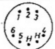
Sockelschaltung
