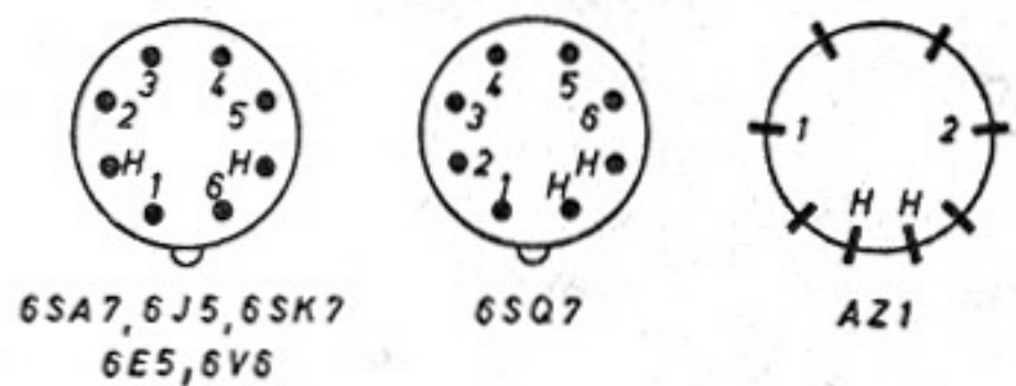
Sockelschaltungen
