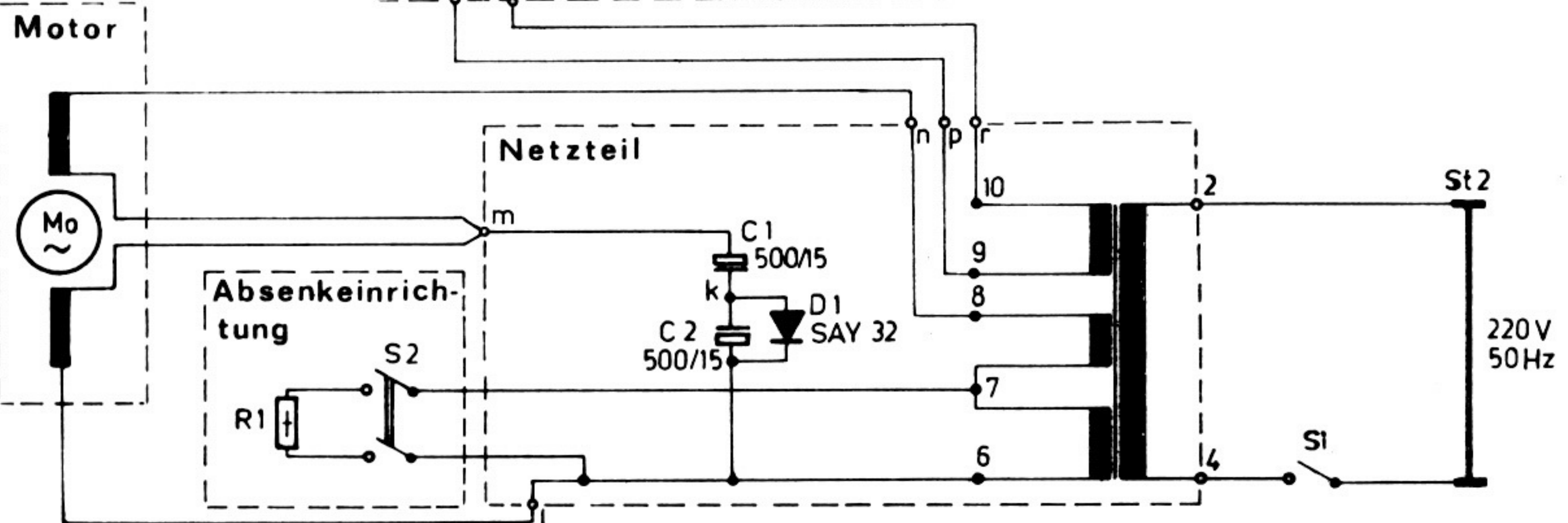
Stromlaufplan ZIPHONA OPAL 216 HiFi Stand 08/73
