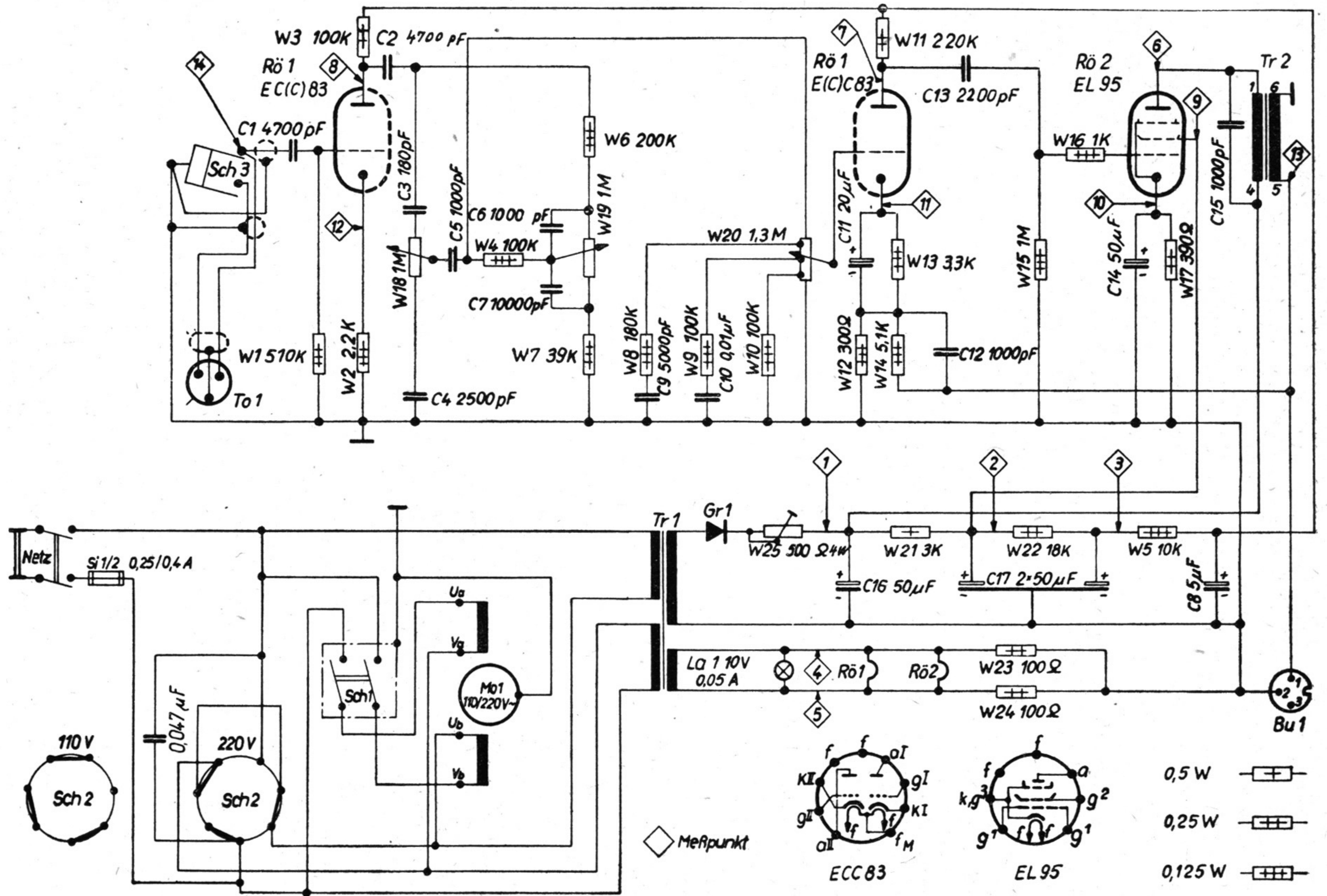
Stromlaufplan Monowiedergabegerät
