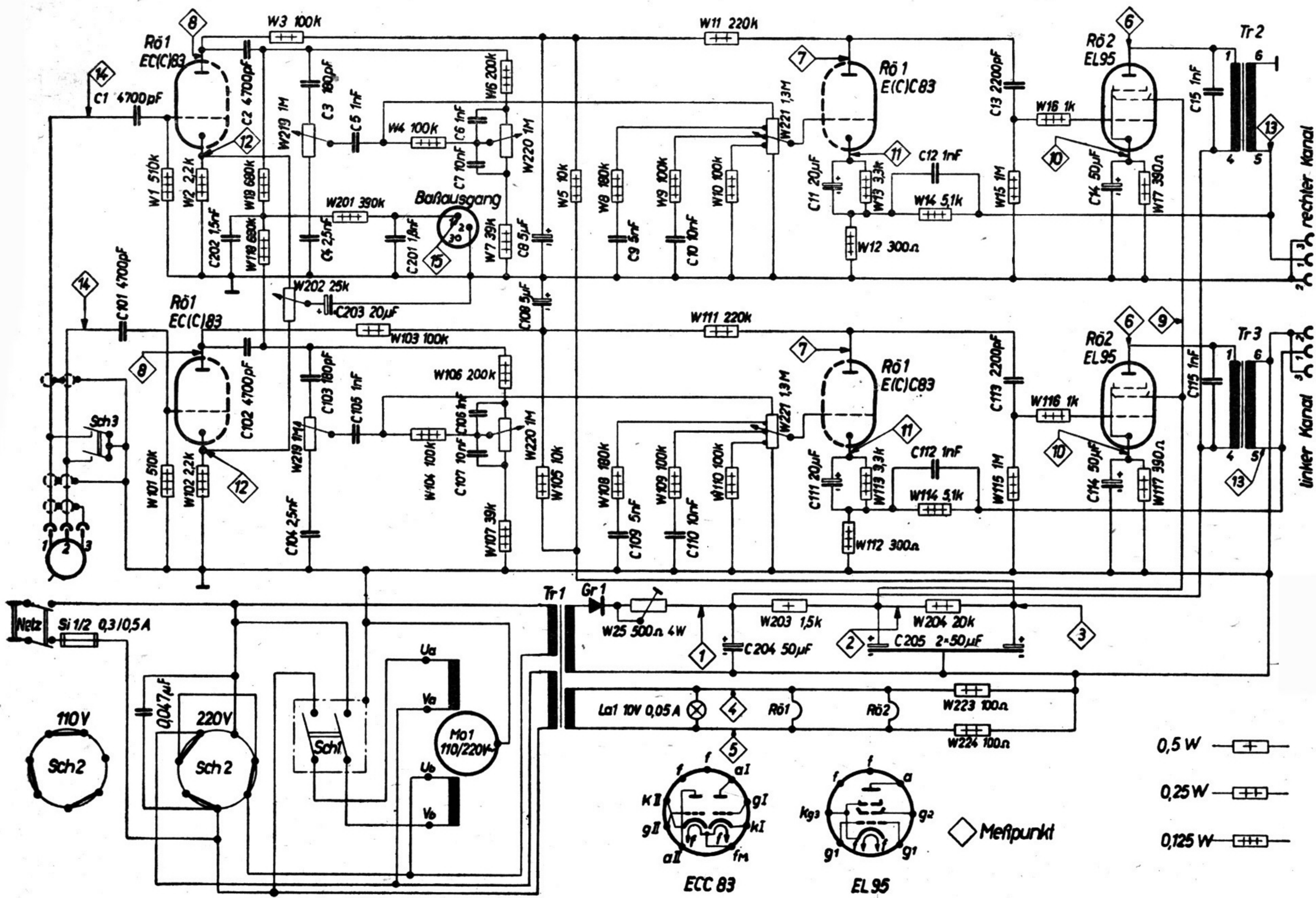
Stromlaufplan Stereowiedergabegerät
