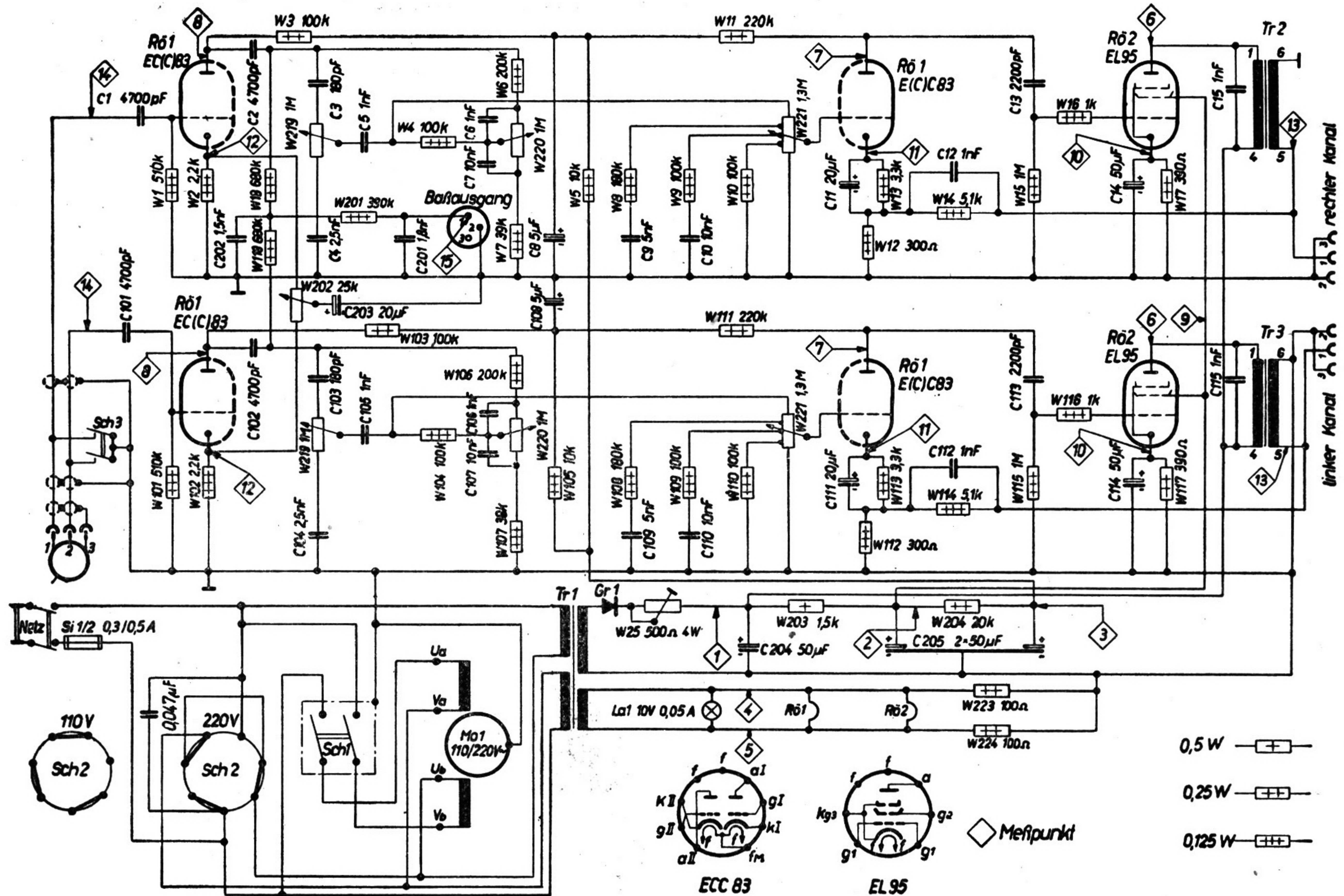
Bild 6 Stromlaufplan P 14-66 KW und P 15-66 KW
