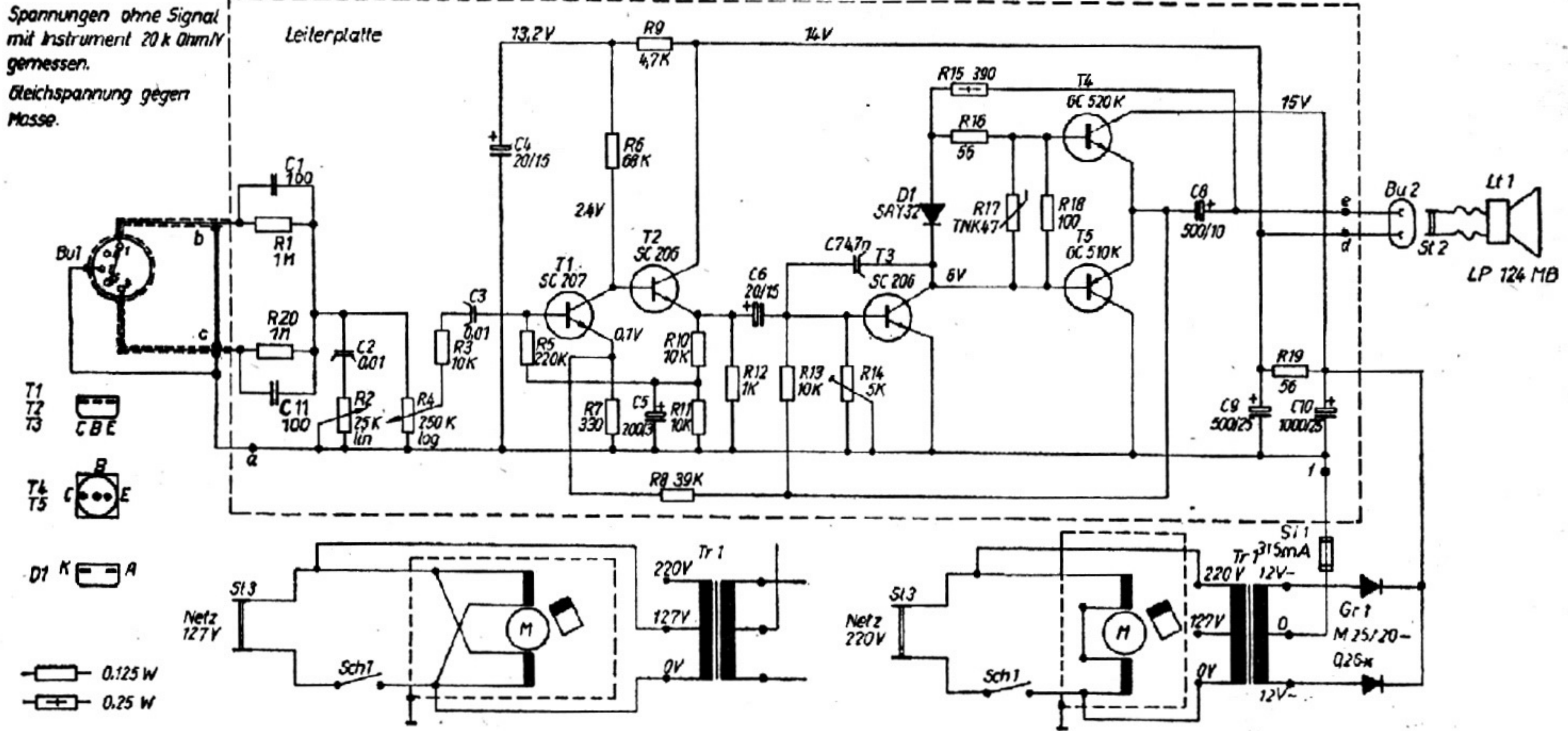
Stromlaufplan Bild 3
