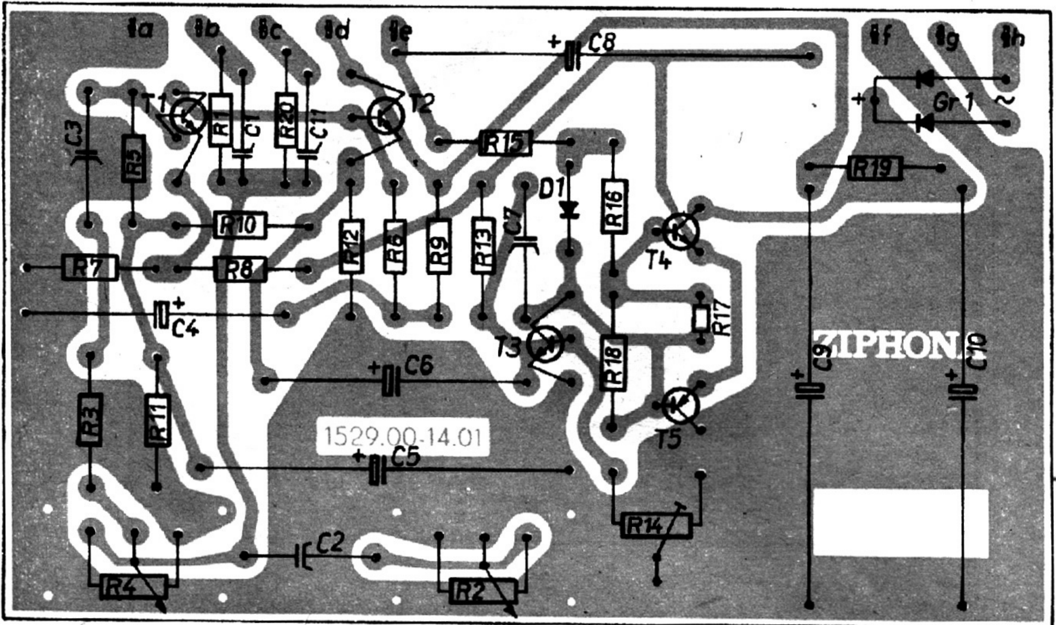
Bild 5 Leiterplatte, verpackt
