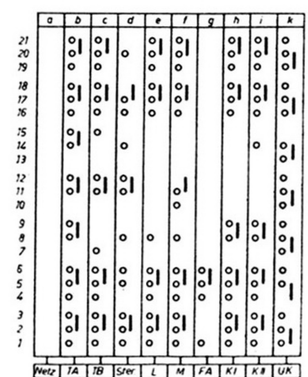
Drucktastenschalter von oben gesehen, UKW gedrückt
