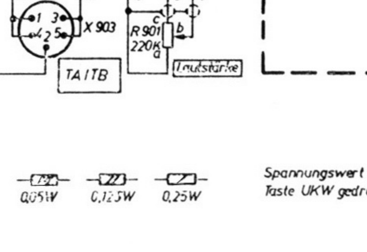
Gezeichnete Schalterstellung keine Taste gedrückt
