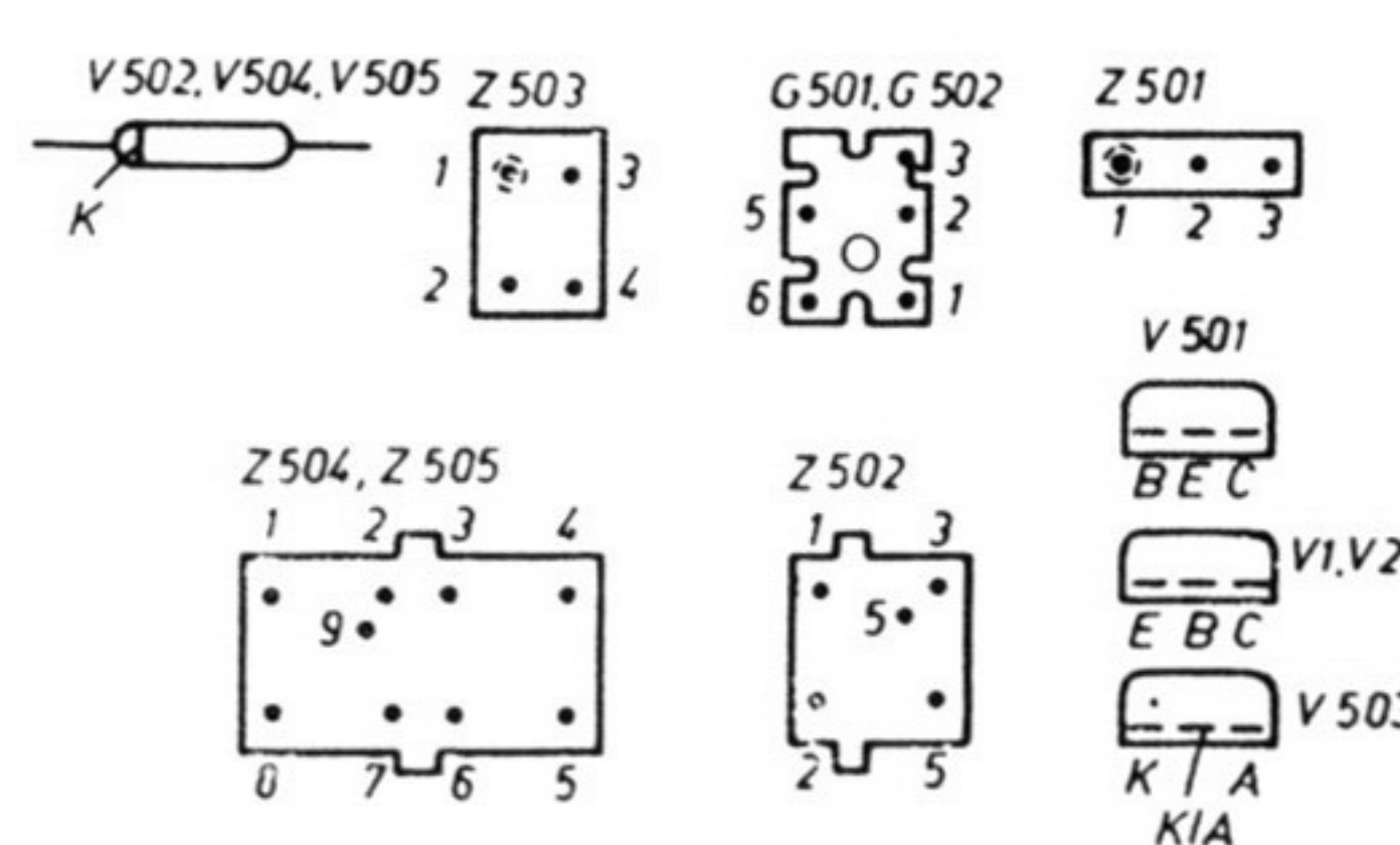
Von unten auf die Anschlüsse gesehen
