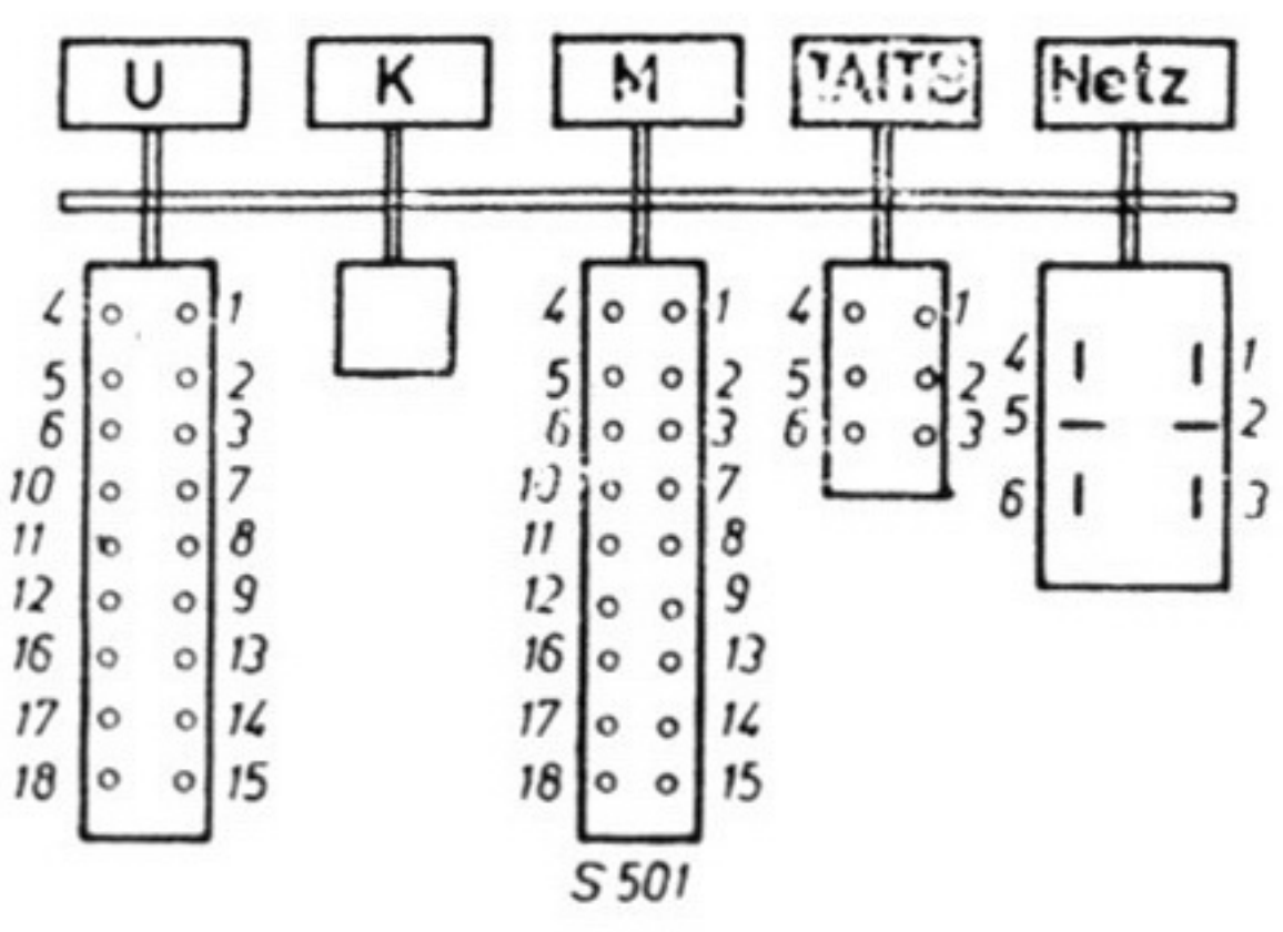
Von oben auf die Lötanschlüsse gesehen
