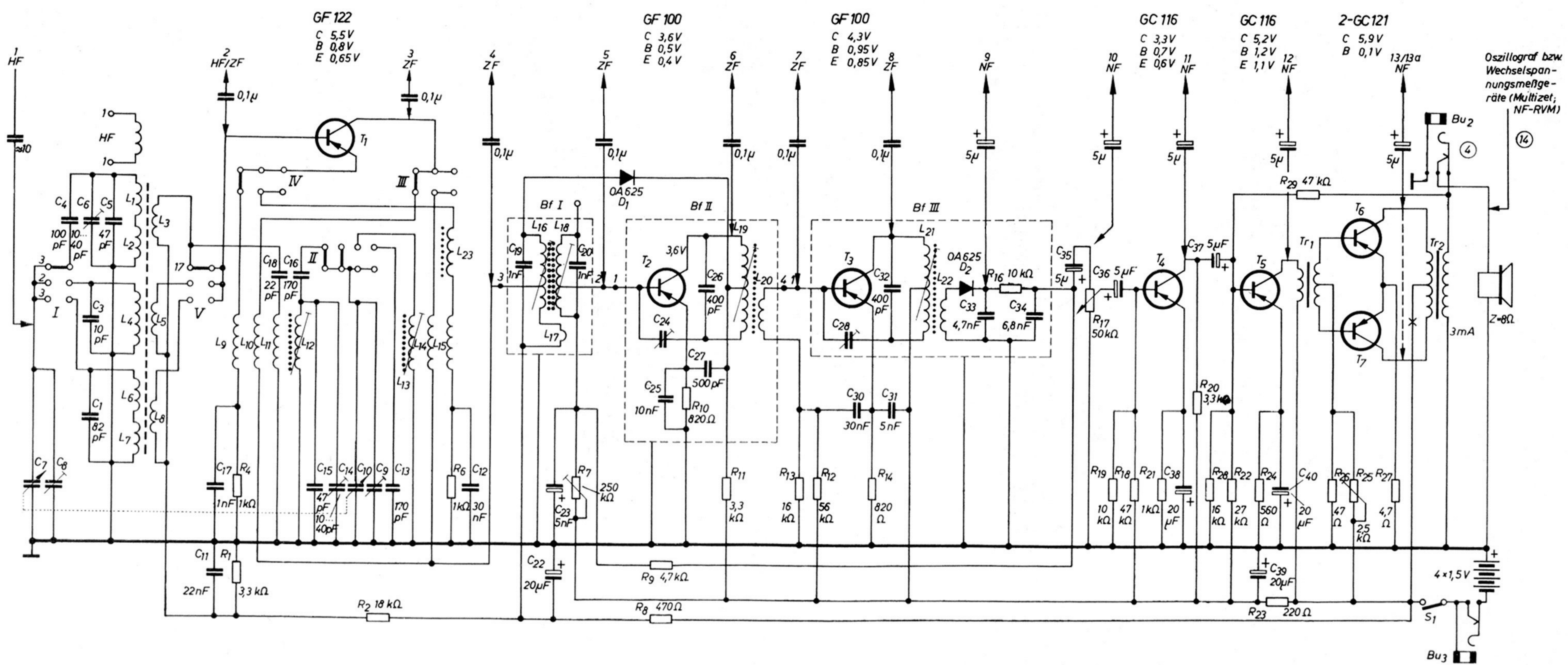
Signalzuführung bzw. -verfolgung beim Taschen-Transistor-Super T 102 (Spannungswerte bei T 3 : C: 5,8 V; B: 1,0 V; E: 0,9 V)
